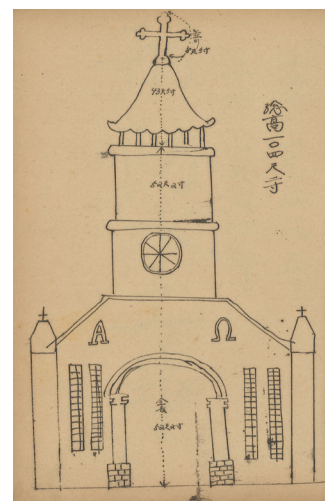
둔율동성당 도면 ▶
